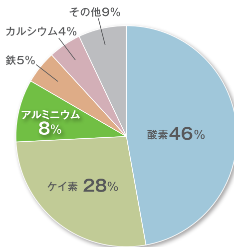
地殻を構成する元素の割合
