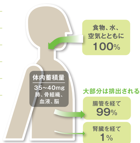
日常生活でのアルミニウムの摂取代謝
